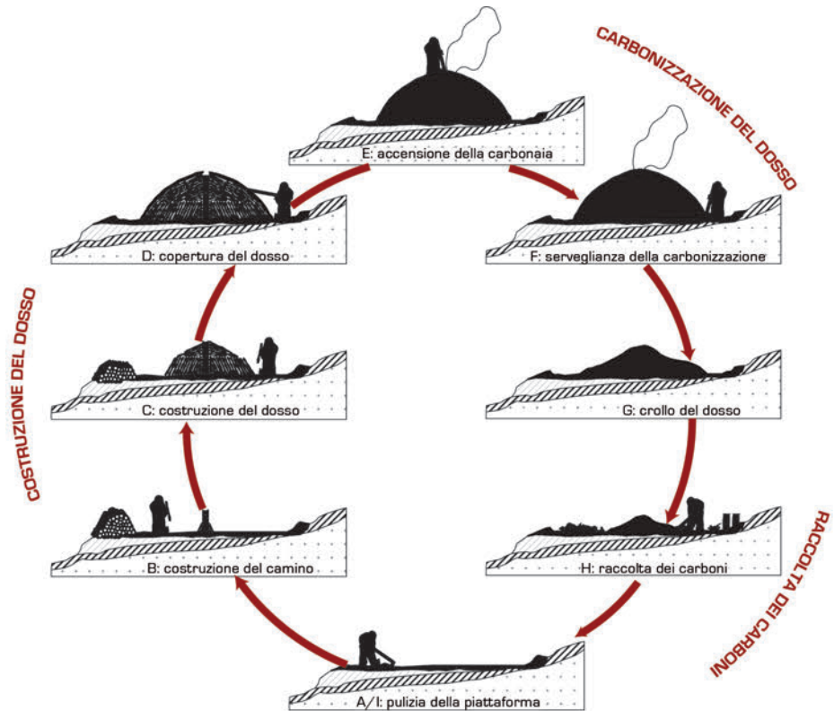
Fig. 6. Funzionamento generale di una carbonaia.
